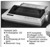
SP-1200 med ekstra udstyr aut. enkeltarkføder.
